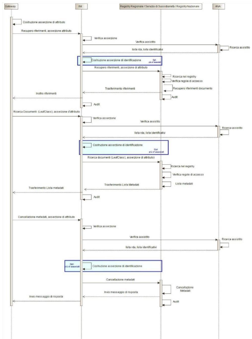
Figura 5 - Scenario 4: Cancellazione logica indice documento
